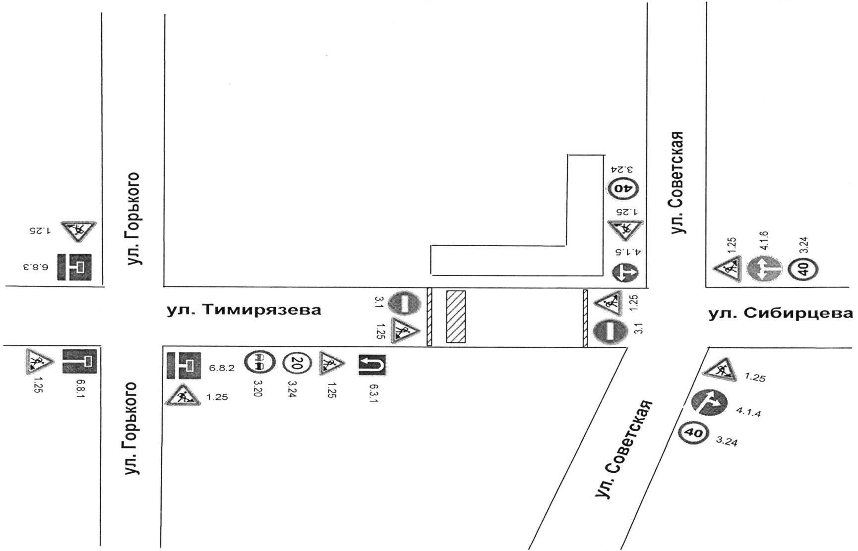
Схема перекрытия места производства работ по адресу ул. Тимирязева в г. Уссурийске.
