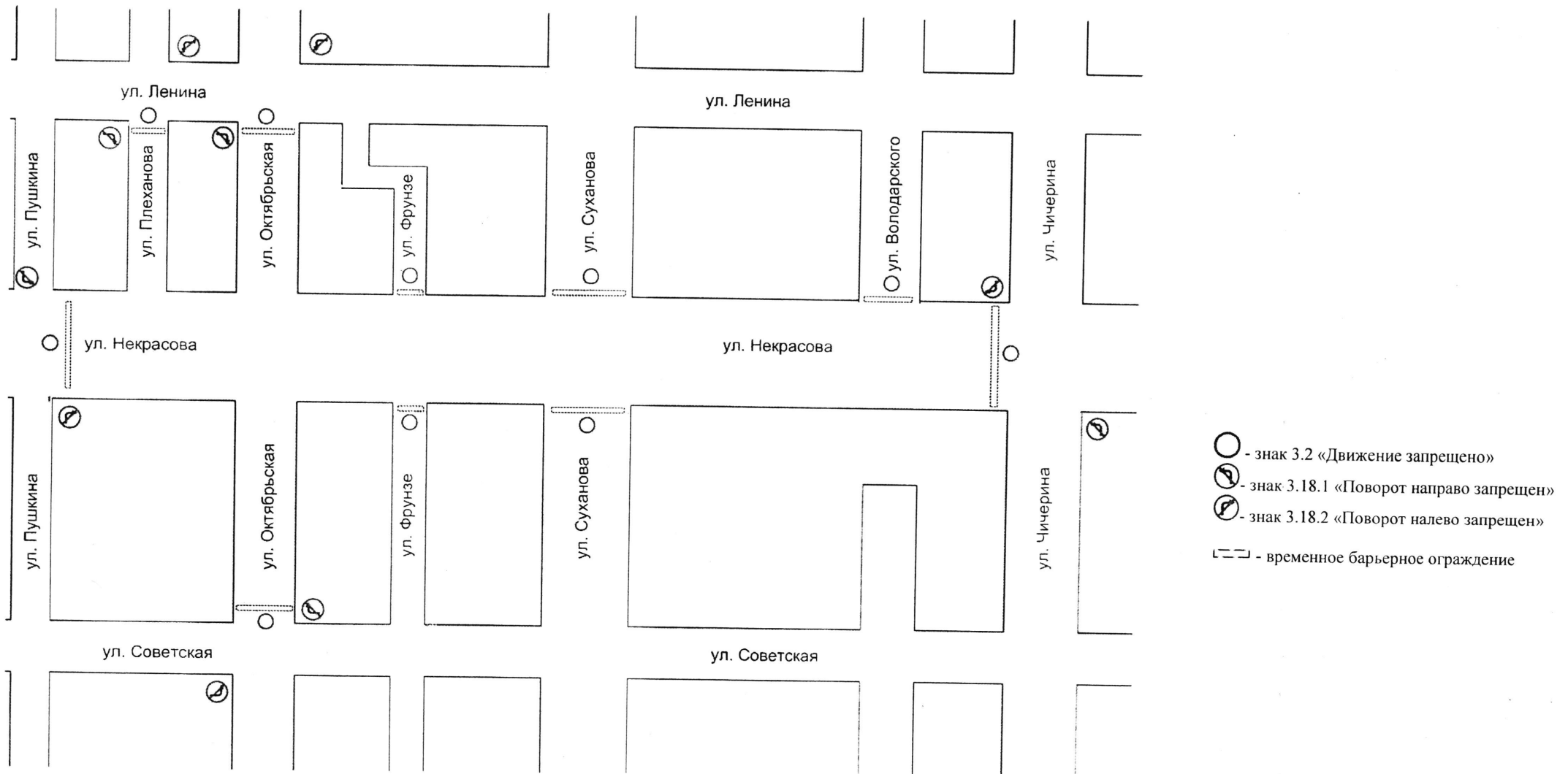
Схема организации перекрытия дорожного движения и маршрутов объезда
